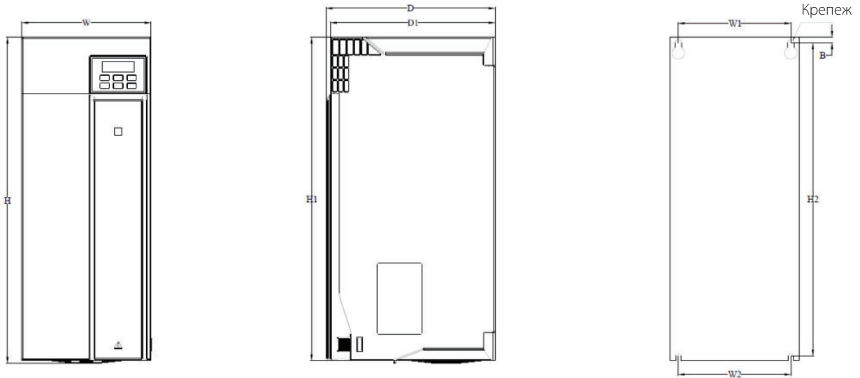
Рис.2-6.5. Чертеж преобразователя частоты типоразмер B5
